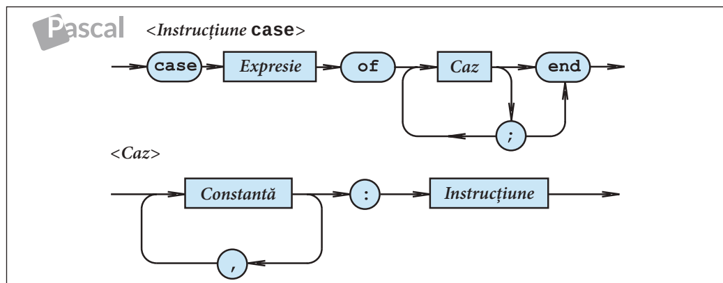
Fig. 3.8. Diagrama sintactică \langle \text{Instrucțiune case} \rangle , PASCAL
