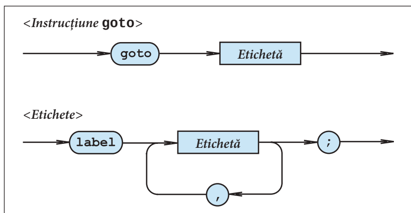
Fig. 3.13. Diagramele sintactice <Instrucțiune goto> și <Etichete>, PASCAL
