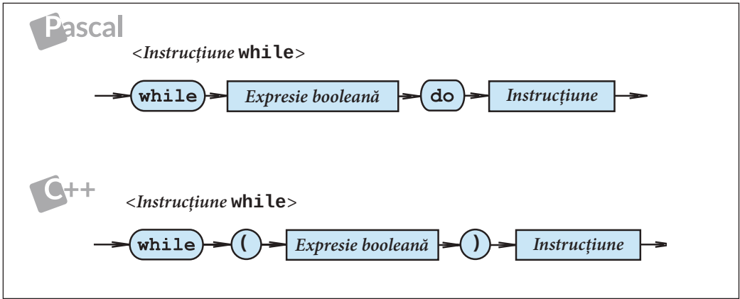
Fig. 3.11. Diagrama sintactică <Instrucțiune while>
