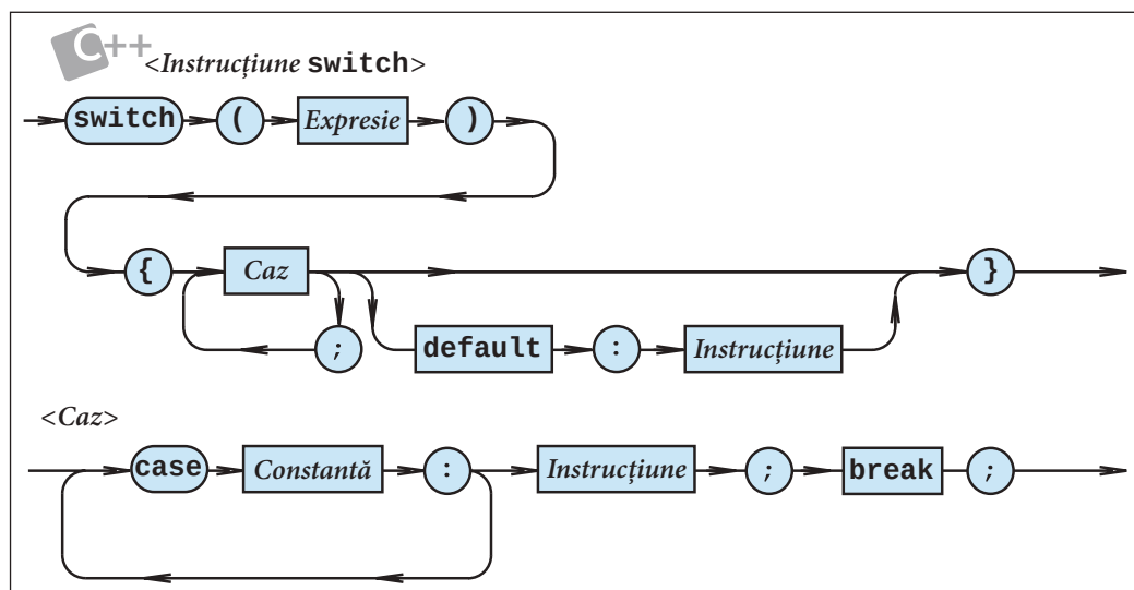
Fig. 3.8*. Diagrama sintactică <Instrucțiune switch>, C++
