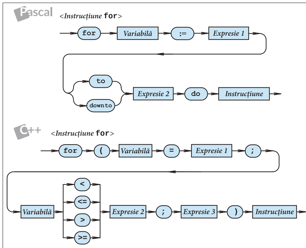
Fig. 3.9. Diagrama sintactică \langle \text{Instrucțiunea for} \rangle
