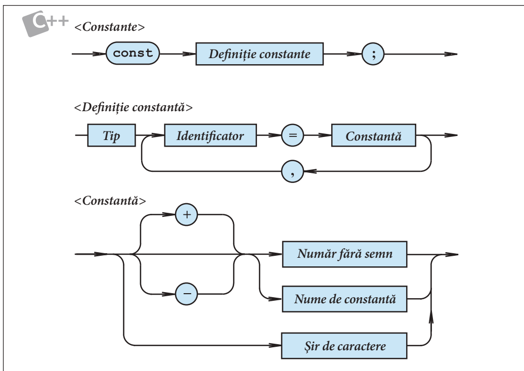
Fig. 2.5.* Diagrammele sintactice <Constante>, <Definiție constantă> și <Constantă>, C++
