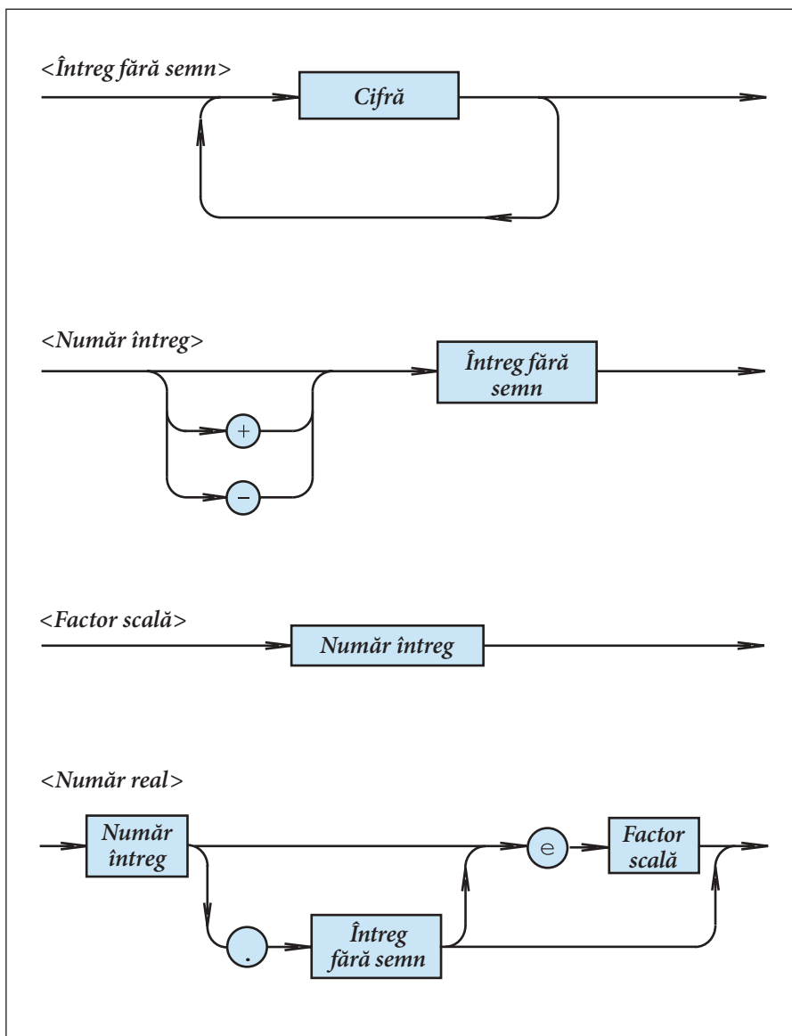
Fig. 1.4. Diagramele sintactice <Număr întreg> și <Număr real>
