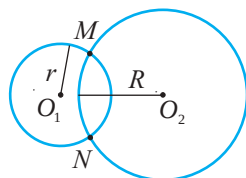
c) secante în punctele M și N
