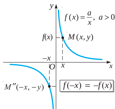
b) Graficul unei funcții impară
