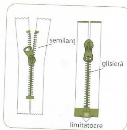
Figura 3.5. Structura fermoarului
