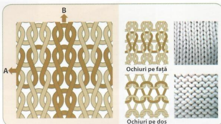
Figura 2.11. Structura tricotelui
