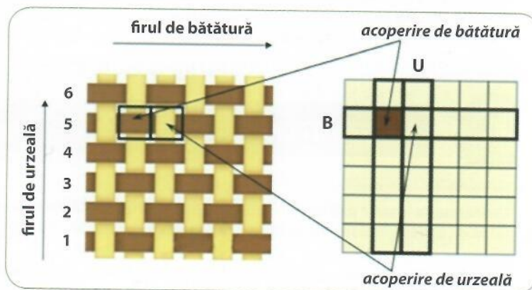
Figura 2.2. Elemente ale țesăturii
