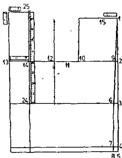
Fig. 8.17. Repartizarea dimensiunilor pentru pensă de bust și răscoiala la gât.
