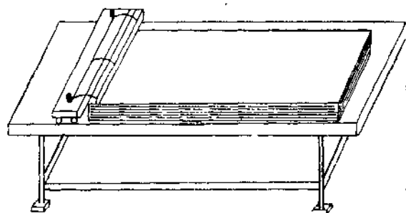
Fig. 4.12. Masa simplă pentru spânuierea manuală.
