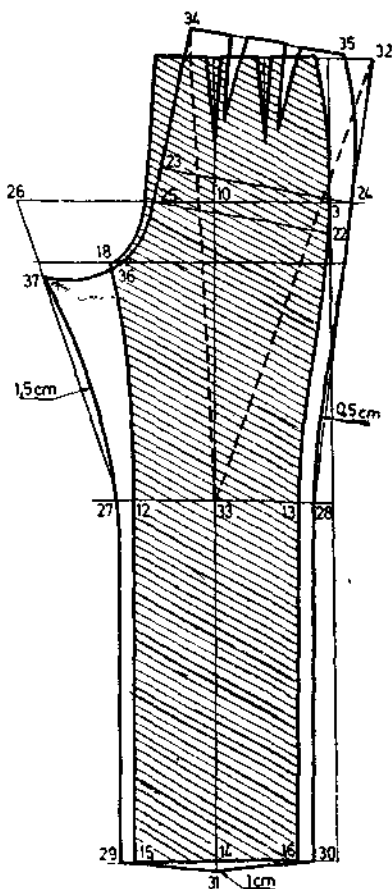
Fig. 8.13. Spate de pantalon.
