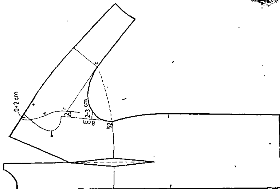
Fig. 8.44. Prelucrarea tiparului de rochie - faşă.
