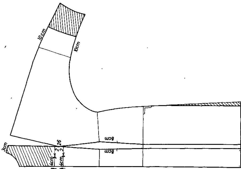
Fig. 8.51. Prelucrarea țiparului pentru față.
