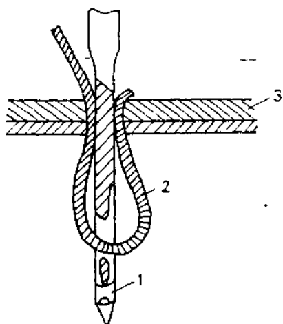
Fig. 4.21. Protejarea aței prin șanțul scurt.
