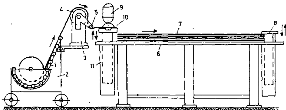
Fig. 4.14. Agregatul pentru spânuierea manual-mecanică.
