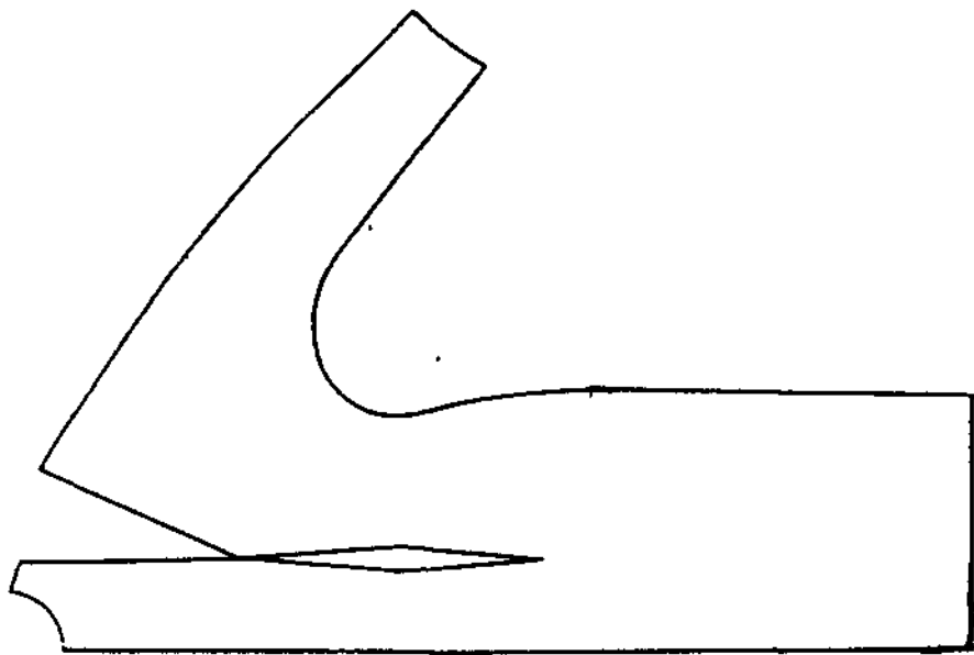
Fig. 8.47. Tipar de rochie chimono – faia – aspect gata.
