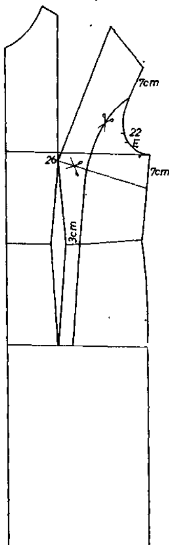
Fig. 8.36. Tiparul de bază al feței.
