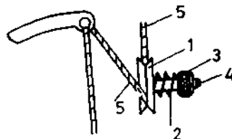
Fig. 4.25. Regulatorul de tensionare a aței.
