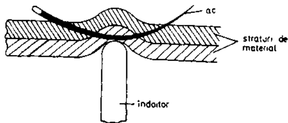
Fig. 4.46. Efectuarea cusăturii ascunse.
