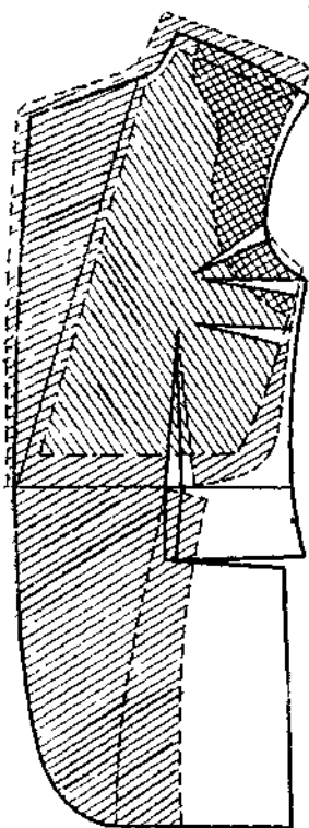
Fig. 10.8. Tipar de întăritură la piepti (sistem)
