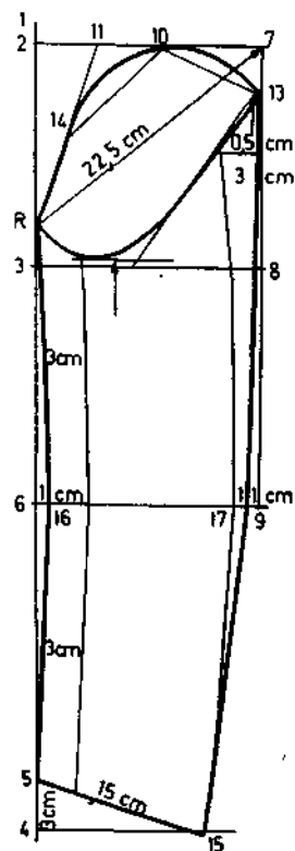
Fig. 8.58. Construirea tiparului de mânecă pentru tajor.
