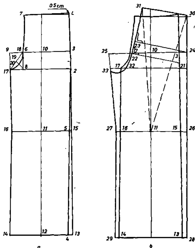
Fig. 8.14. Pantaloni încrețit în talie.
