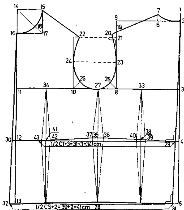
Fig. 9.5. Construcţia tiparului de bluză.
