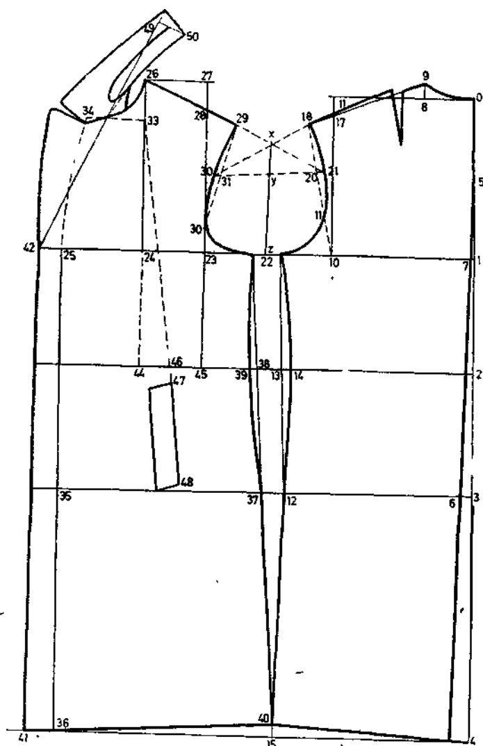
Fig. 10.23. Tipar de pardesiu impermeabil.
