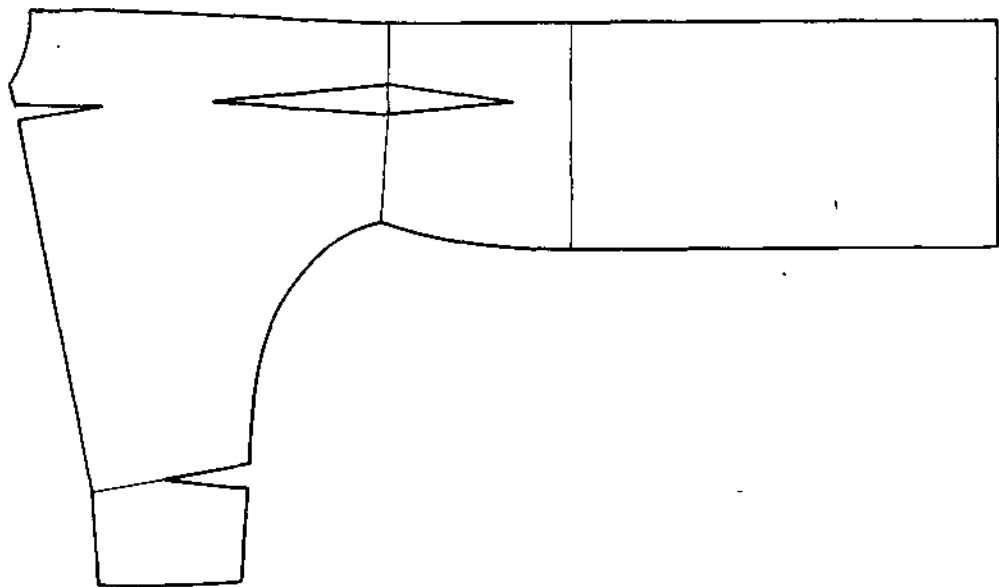
Fig. 8.50. Aspectul final al tiparului de spat.
