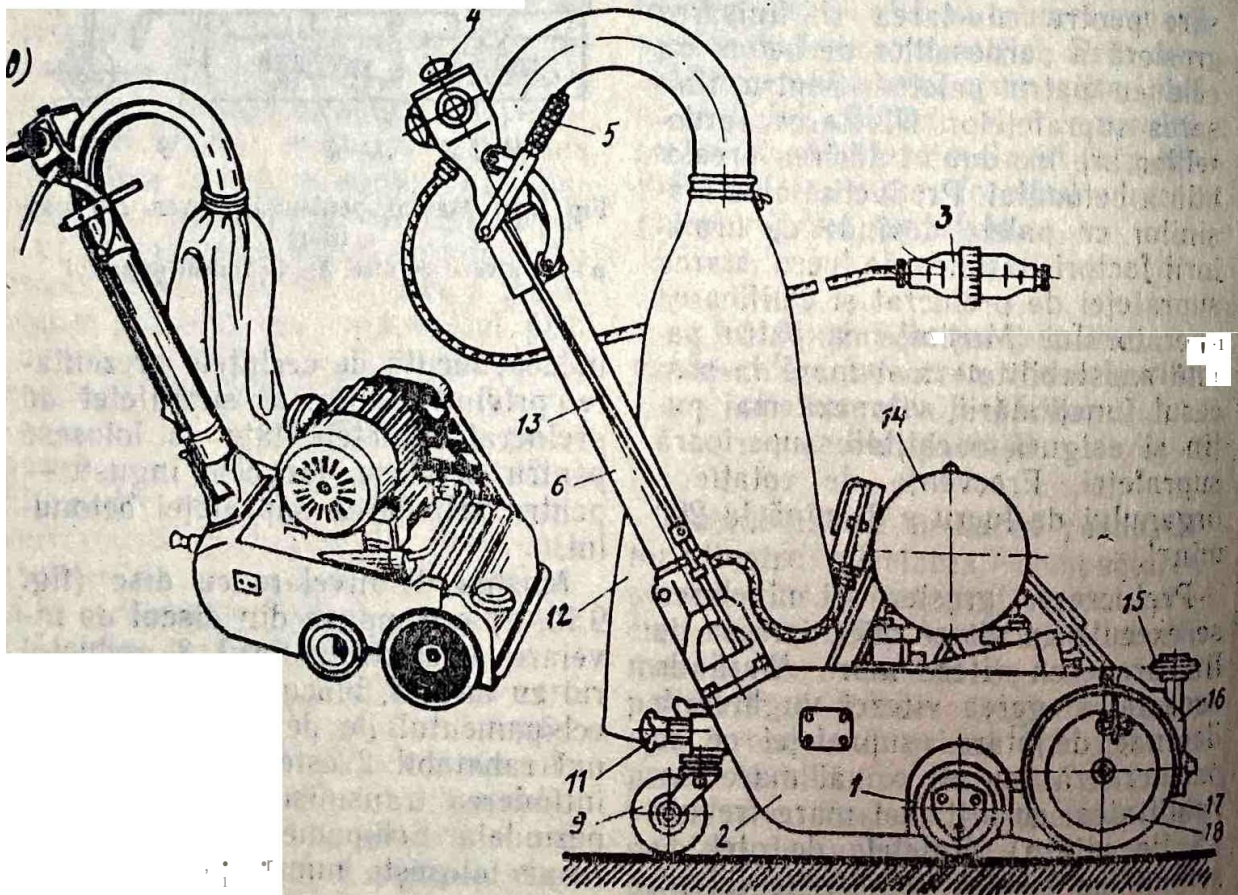
Fig. 9.11. Mașini pentru prelucrarea pardosimilor: a- de roșchetat; b- de lustruit
